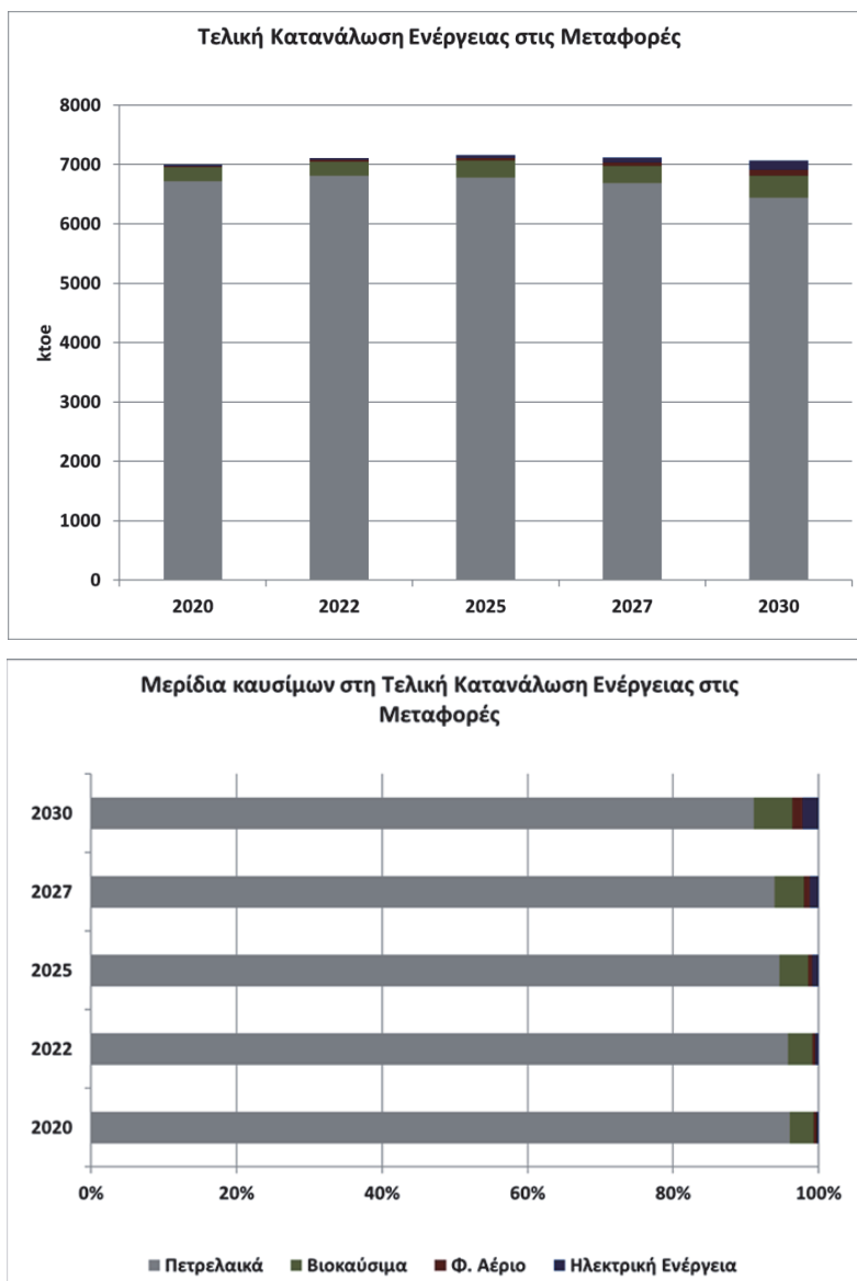
Διάγραμμα 42: Εξέλιξη τελικής κατανάλωσης ενέργειας στον τομέα των μεταφορών έως το έτος 2030.
