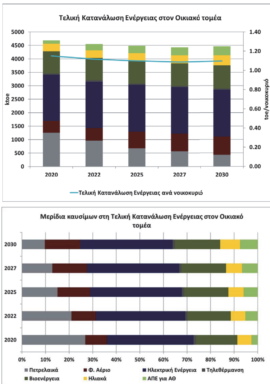
Διάγραμμα 40: Εξέλιξη τελικής κατανάλωσης ενέργειας στον οικιακό τομέα έως το έτος 2030.
