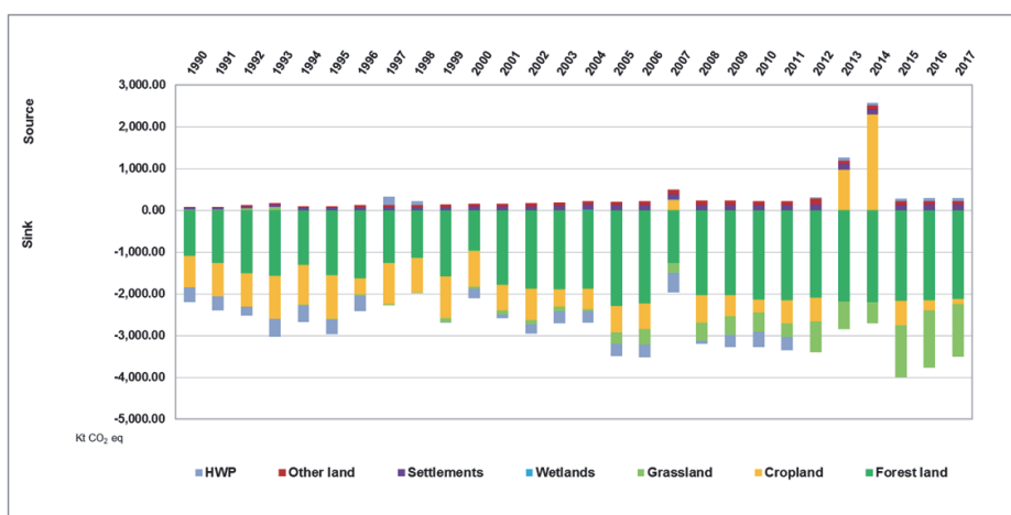
Διάγραμμα Β.3: Καθαρές εκπομπές/απορροφήσεις GHG (σε ktCO 2 eq) από τον τομέα LULUCF ανά κατηγορία χρήσεων γης για την περίοδο 1990-2017 (πηγή: 2019 Ετήσια Εθνική Απογραφή GHG στην UNFCCC)
